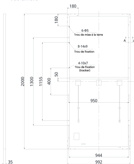
Vue arrière
