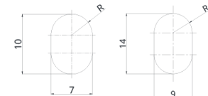
Trous de fixation
