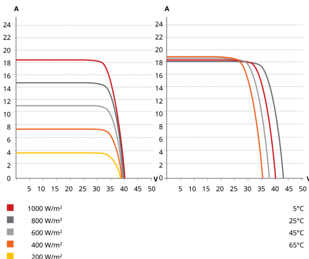
COURBES DE FAIBLES ÉCLAIREMENTS ET DE TEMPÉRATURES
